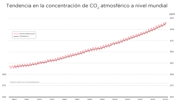
Figura 11. Tendencia en la concentración de CO 2 atmosférico a nivel mundial. Fuente: https://www.unenvironment.org/es/noticias-y-reportajes/reportajes/el-mundo-registra-concentracion-record-de-dioxido-de-carbono-pesar
